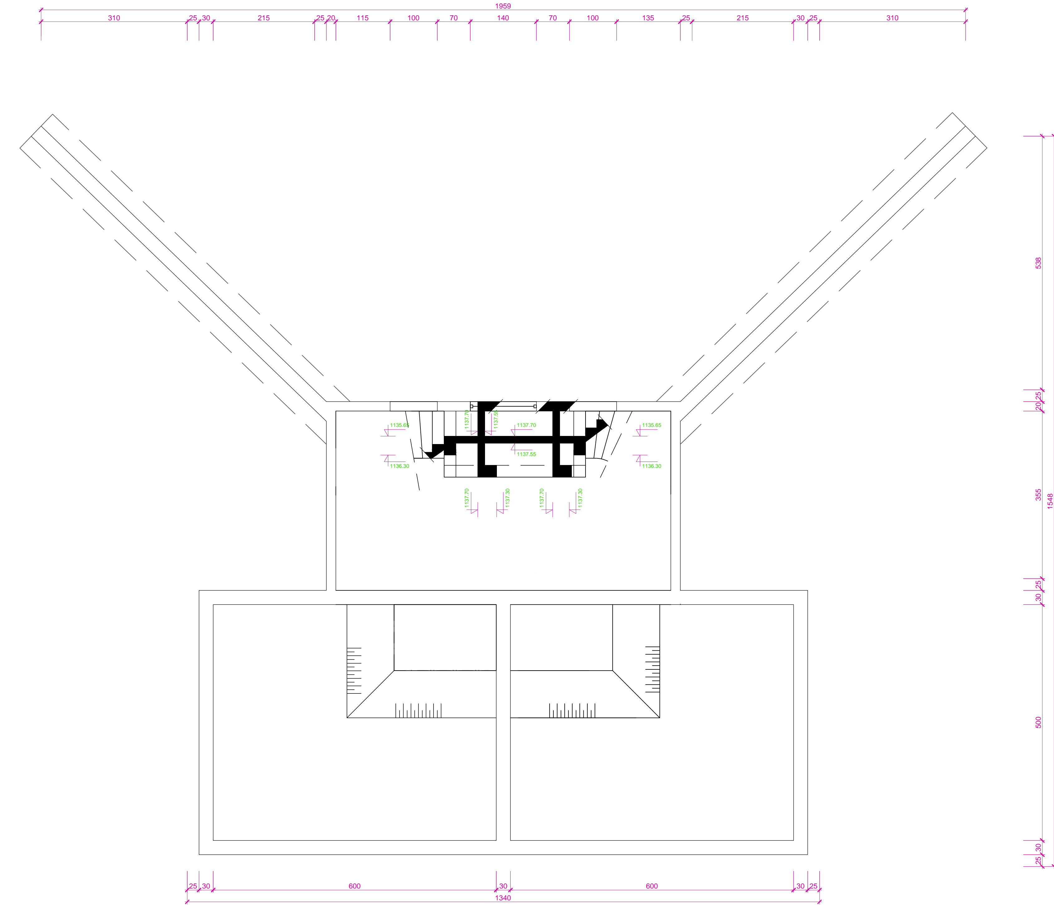
NACRT OPLATE TEMELJNE PLOČE NA KOTI : 1137.70
