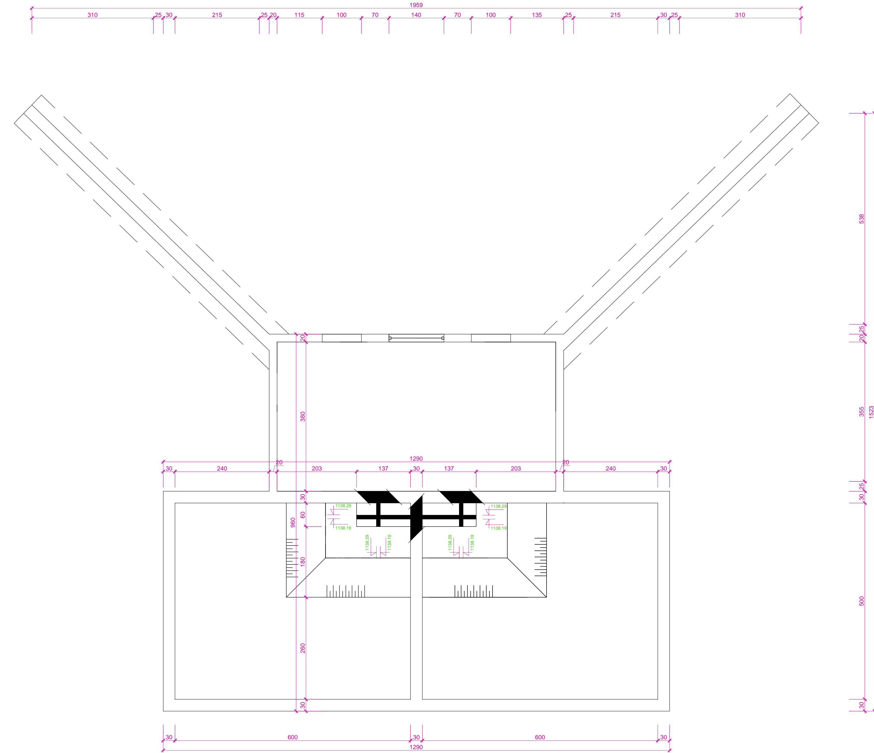
NACRT OPLATE TEMELJNE PLOČE NA KOTI : 1138.29
