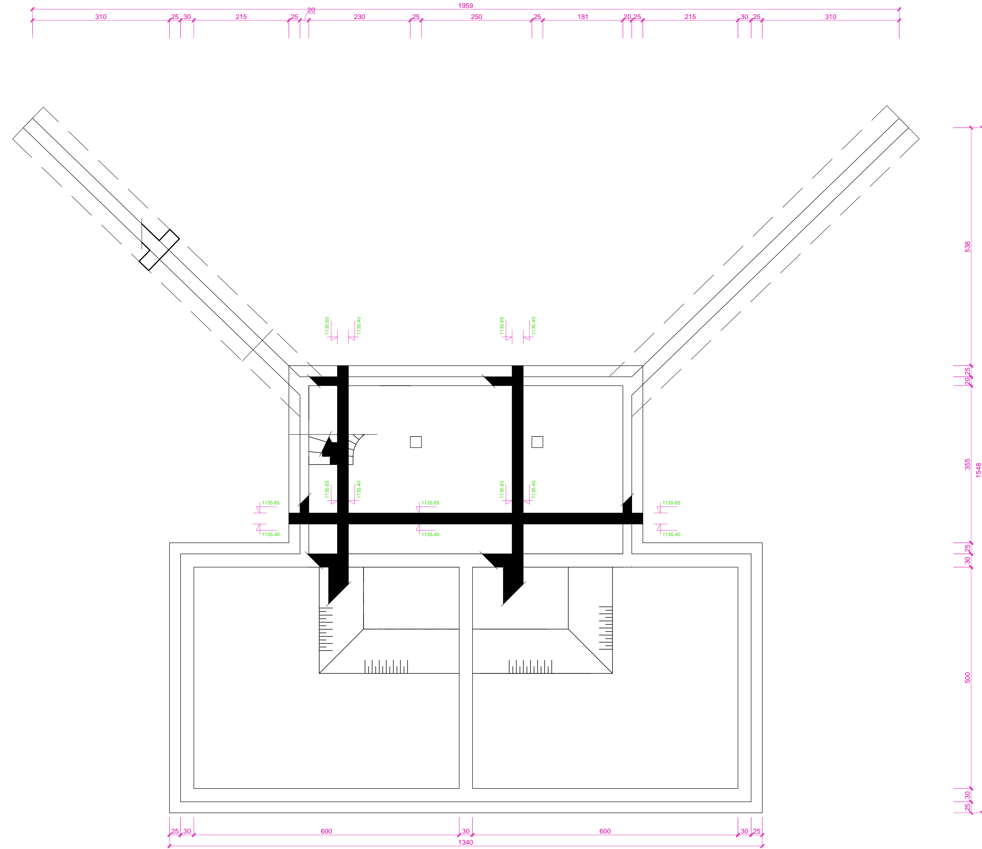
NACRT OPLATE TEMELJNE PLOČE NA KOTI : 1135.65
