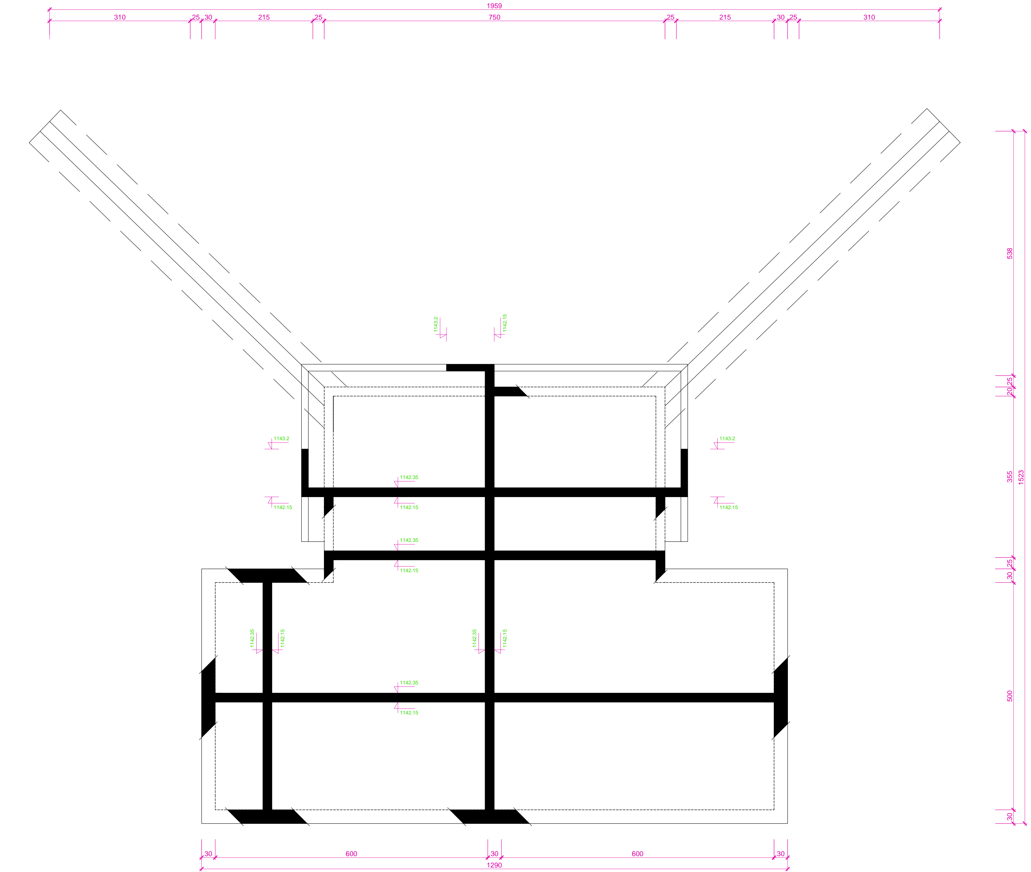
NACRT OPLATE TEMELJNE PLOČE NA KOTI : 1142.35
