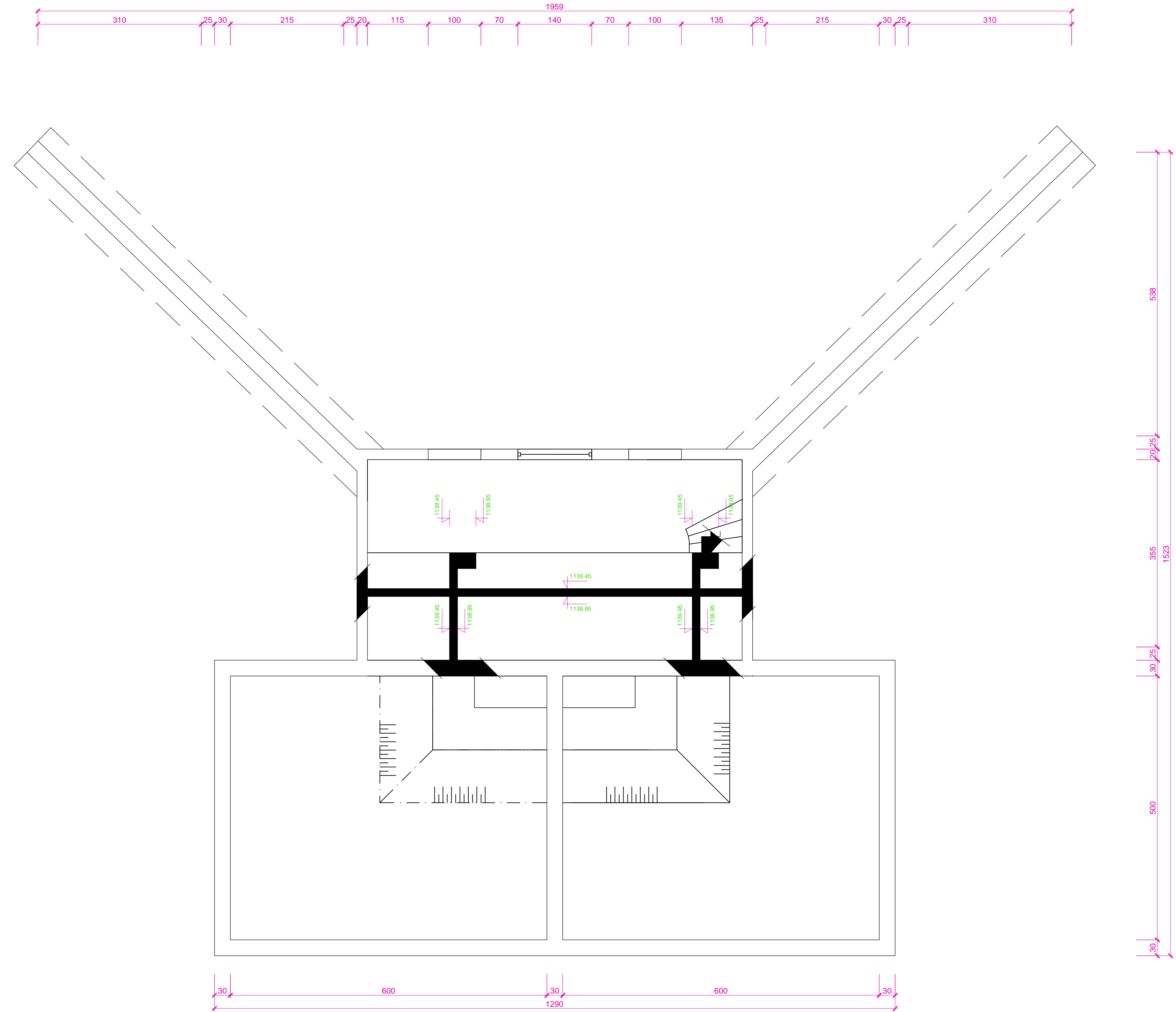
NACRT OPLATE TEMELJNE PLOČE NA KOTI : 1139.45
